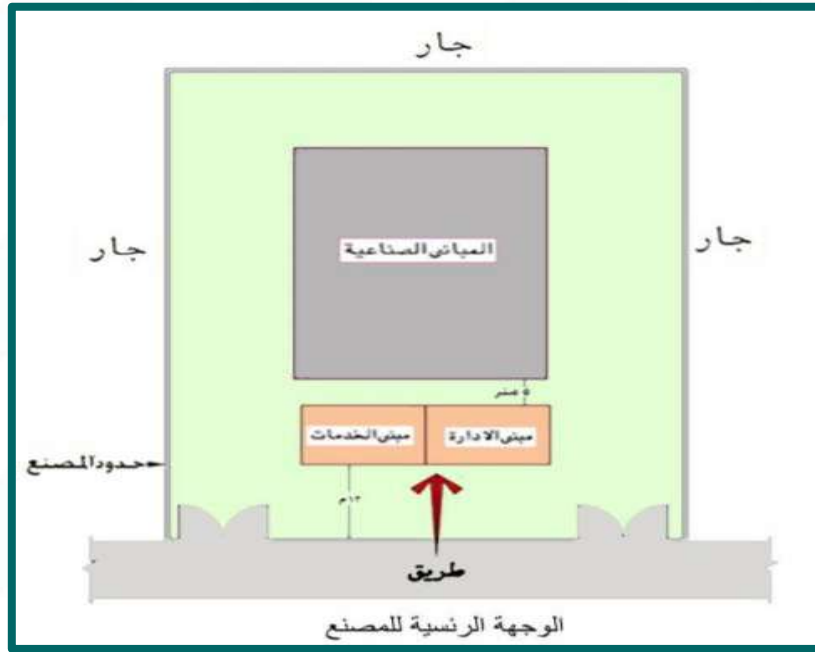
شكل رقم (5) يوضح موقع مبنى الإدارة وخدمات العاملين
